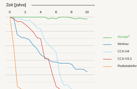
Zersetzungsraten von Bodenpfählen [Zustandsindex]
