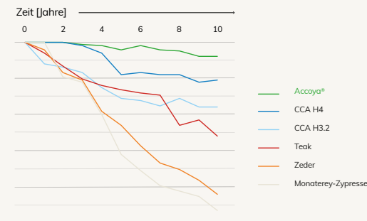
Zersetzungsraten von Bodenpfählen [Zustandsindex]
